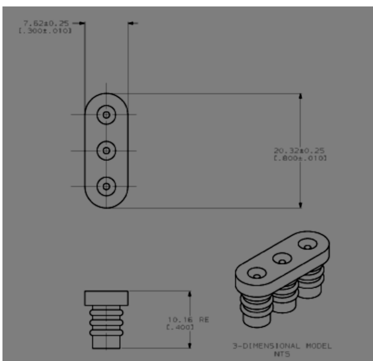
Selo de vedação (wire seal)
