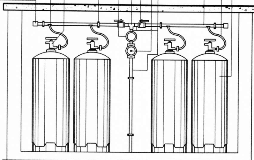
CORTE BB
