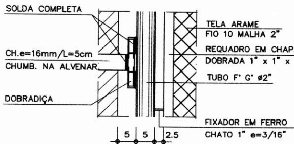
DETALHE 1 - DOBRADIÇA ESCALA 1:10
