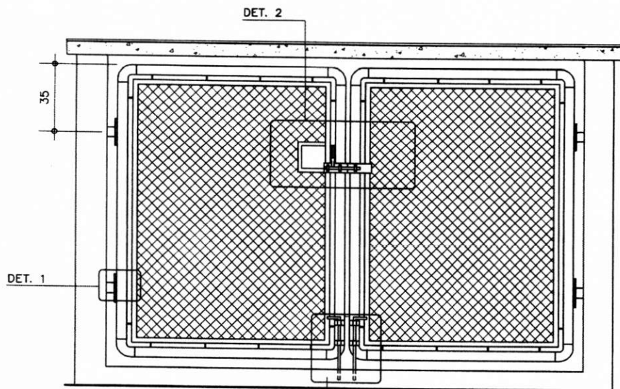
VISTA A
