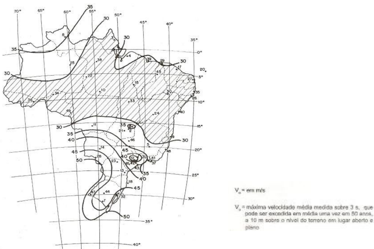
Velocidade básica do vento, mapa apresentado pela NBR 6123 (ABNT, 1988, p.6)
