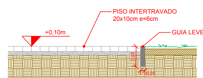
DETALHAMENTO DO PISO INTERTRAVADO ESC 1:25
